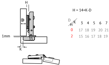
dobradiça amortecedor C26 reta 01.06.510 R
