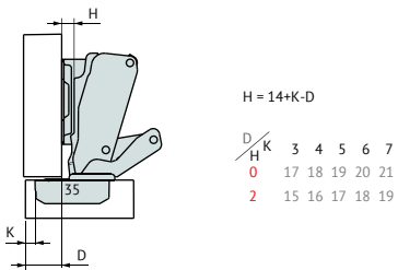
dobradiça 30° negativos C35 01.06.503
