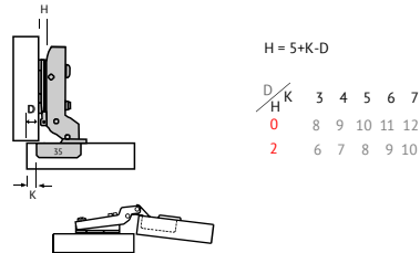
dobradiça 180° C35 meia-curva 01.06.511 M
