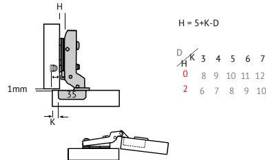
dobradiça amortecedor C26 meia curva 01.06.510 M
