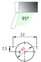
dobradiça amortecedor C40 curva total 01.06.501 C
