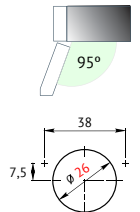
dobradiça amortecedor C26 curva total 01.06.510 C
