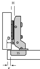
dobradiça mola C40 meia-curva 01.06.514 M
