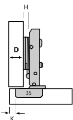
dobradiça mola C40 reta 01.06.514 R
