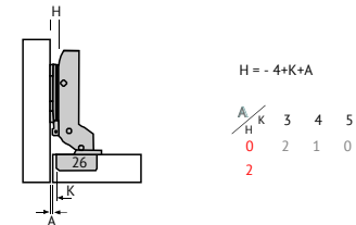
dobradiça amortecedor C40 curva total 01.06.501 C
