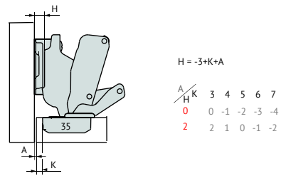
dobradiça 90° rabo curto C35 reta 01.06.512 R
