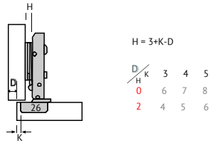
dobradiça amortecedor C40 meia-curva 01.06.501 M
