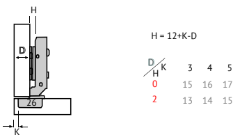
dobradiça amortecedor C40 reta 01.06.501 R
