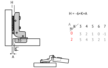
dobradiça amortecedor C26 curva total 01.06.510 C
